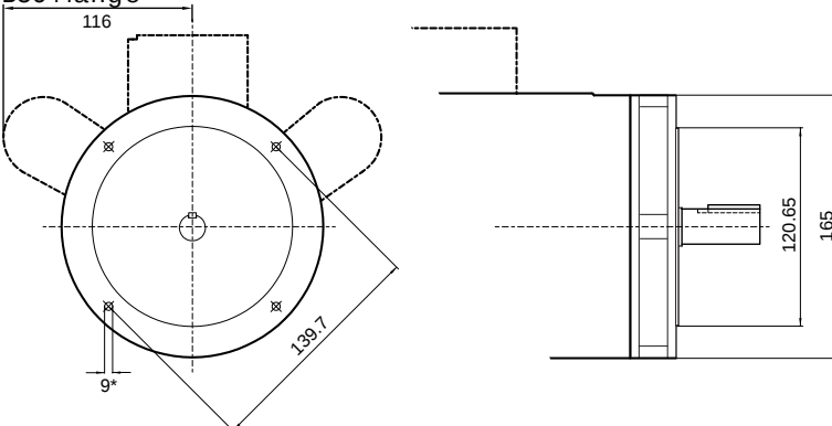
B56 Flange
